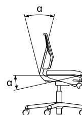
Mécanisme synchrone « Freefloat » avec dispositif de blocage
